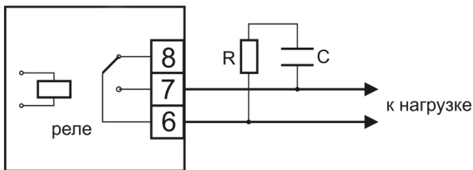
Рисунок 3.8 Подключение нагрузки к релейному выходу
