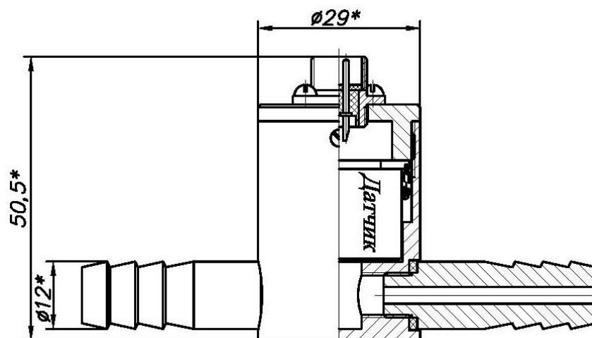
Рисунок 3.11 Преобразователь ИПК-02
