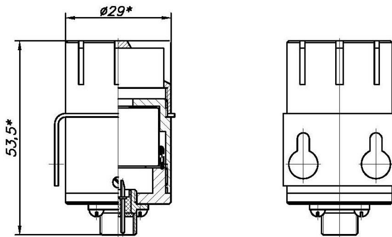
Рисунок 3.10 Преобразователь ИПК-01
