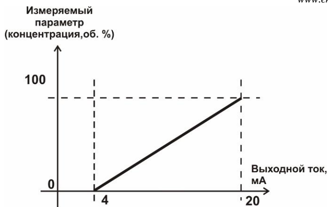
Рисунок 3.9 Линейный выход 4...20 мА по концентрации кислорода от 0 до 100 об. %
