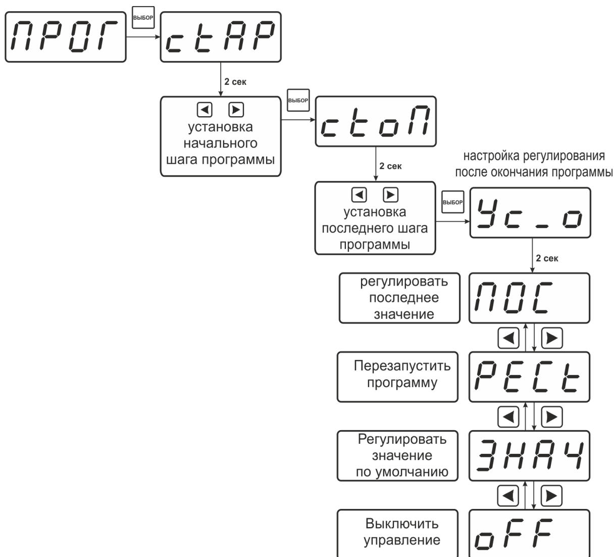
Рисунок 6.19 Схема настройки программы
