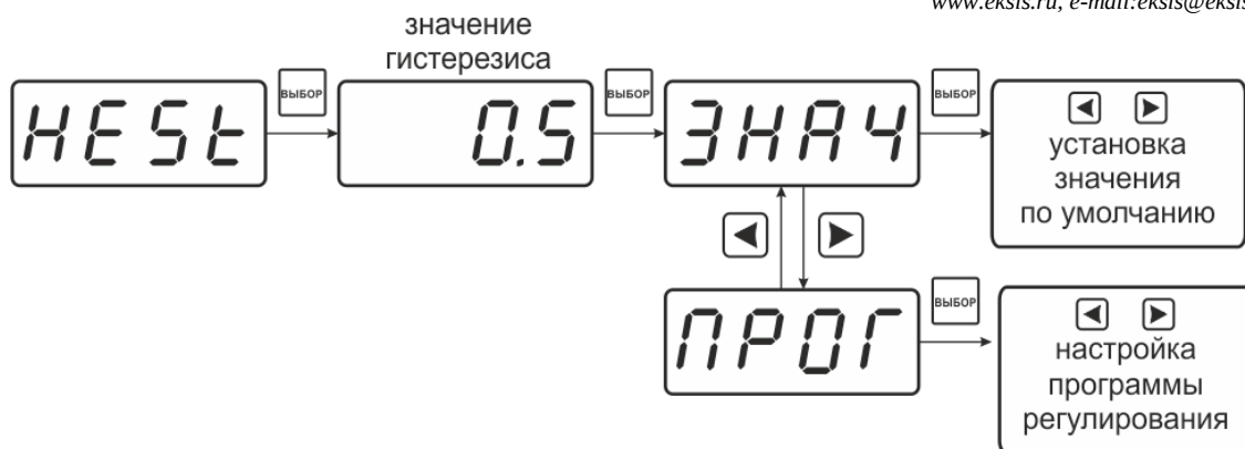
Рисунок 6.18 Задание величины гистерезиса
