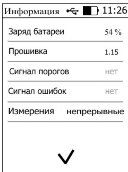
Рисунок 5.7 Меню «Информация»
