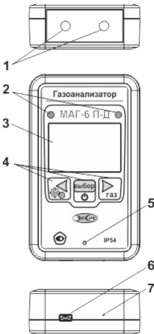
Рисунок 3.1 Переносной многокомпонентный газоанализатор МАГ-6 П-Д(-В)
