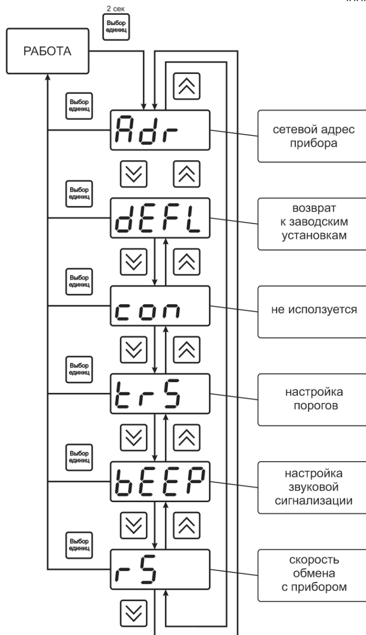
Рисунок 6.4 Режим “Настройка”
