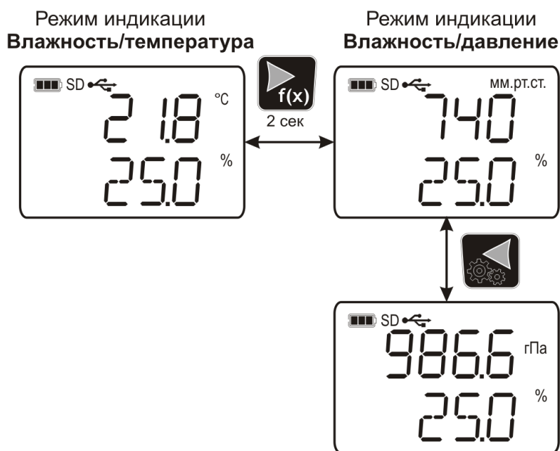
Рисунок 5.2 Переключение режимов индикации ИВТМ-7 К-Д-1
