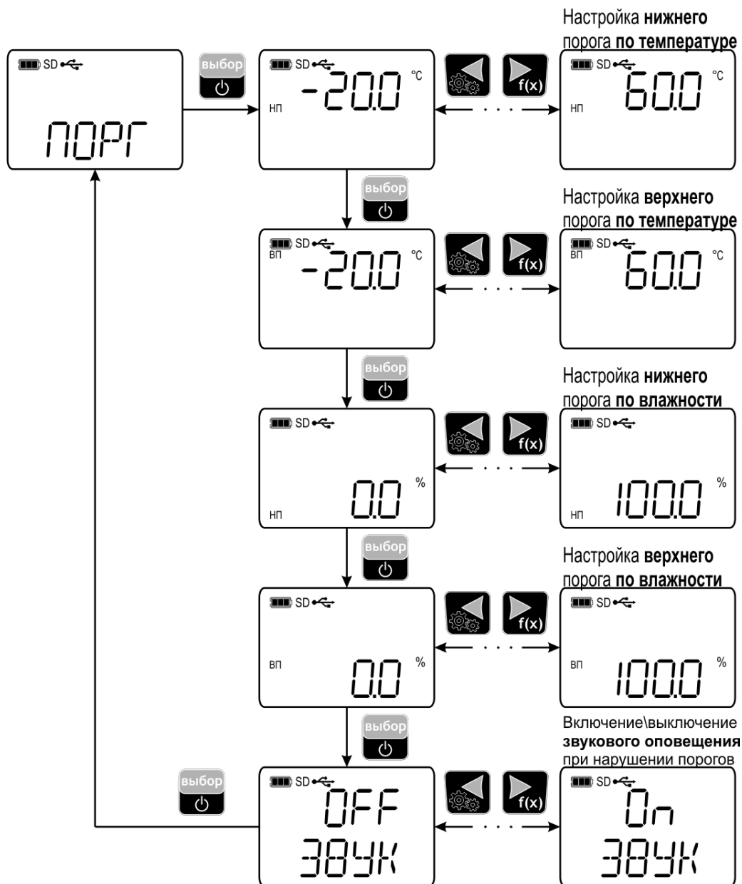
Рисунок 5.4 Установка порогов
