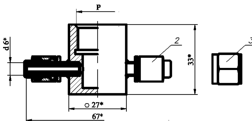
Рисунок В2– Проточная камера со штуцерами d=6
