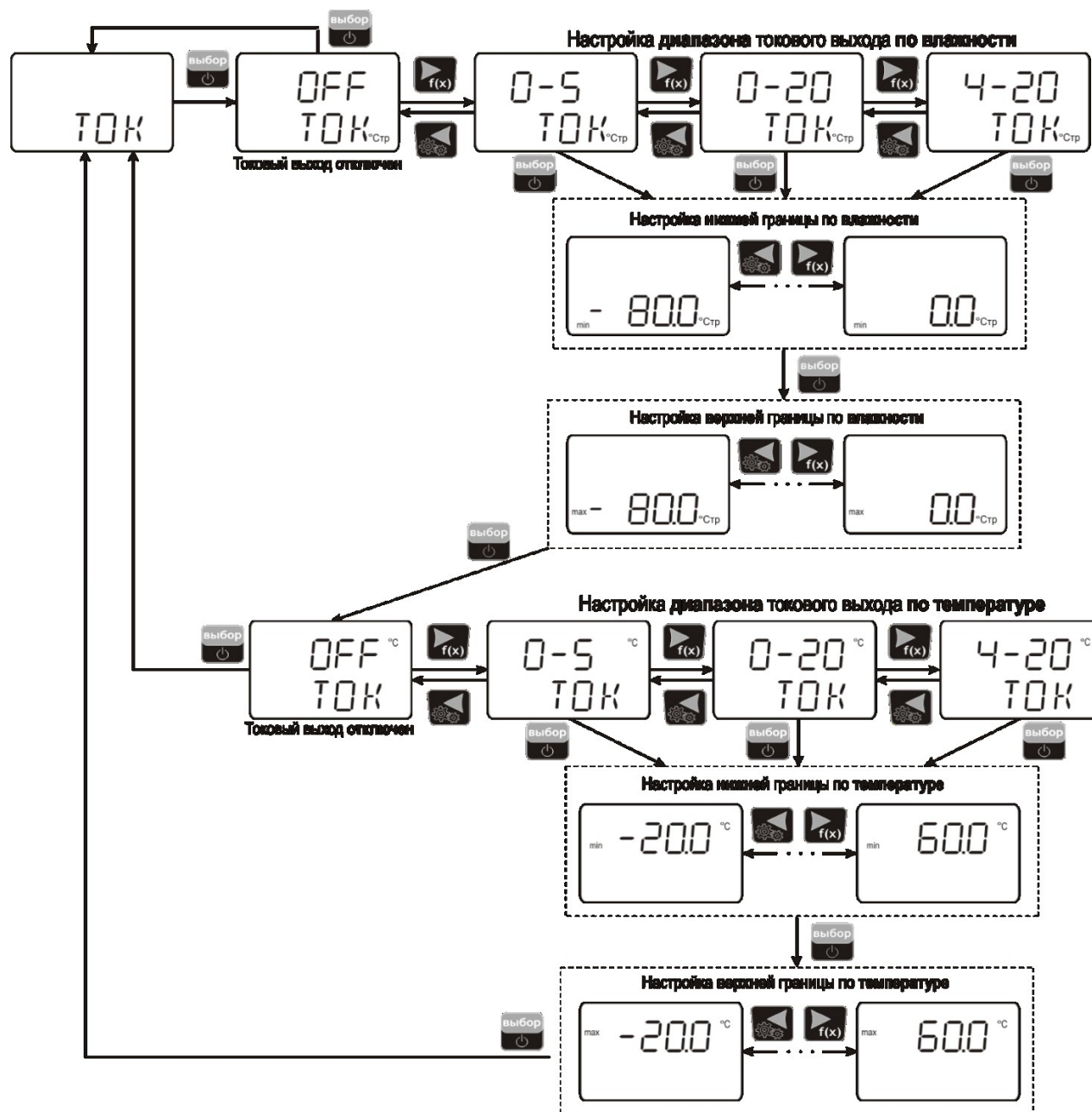
Рисунок 5.4–Настройка токовых выходов
