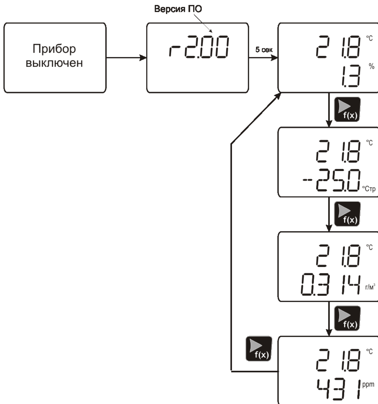
Рисунок 5.1–Режим «РАБОТА»
