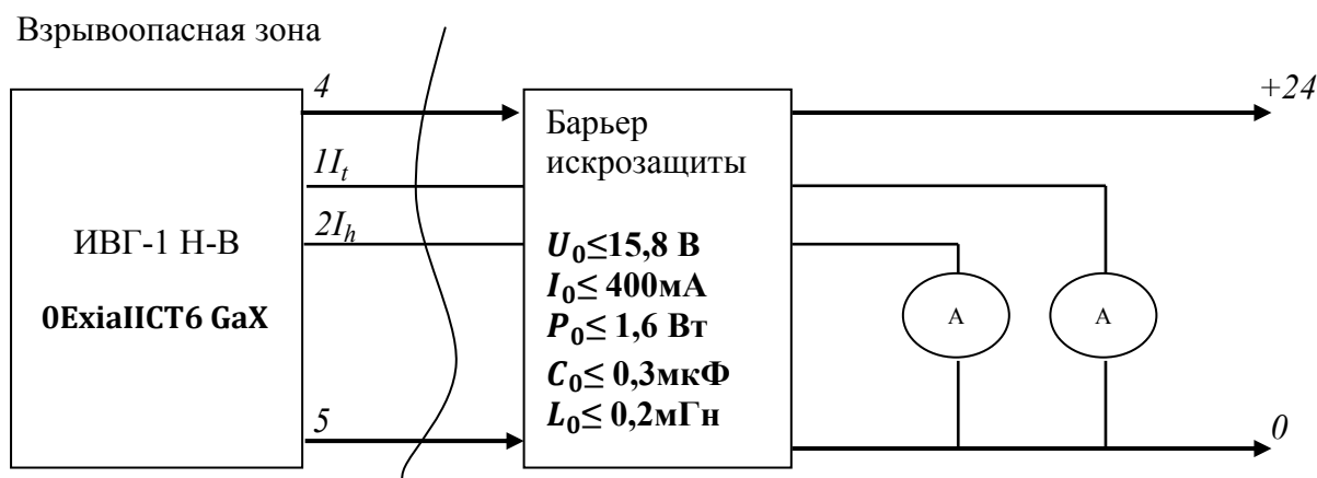
Рисунок 4.1–Схема подключения ИВГ-1 Н-(В)
