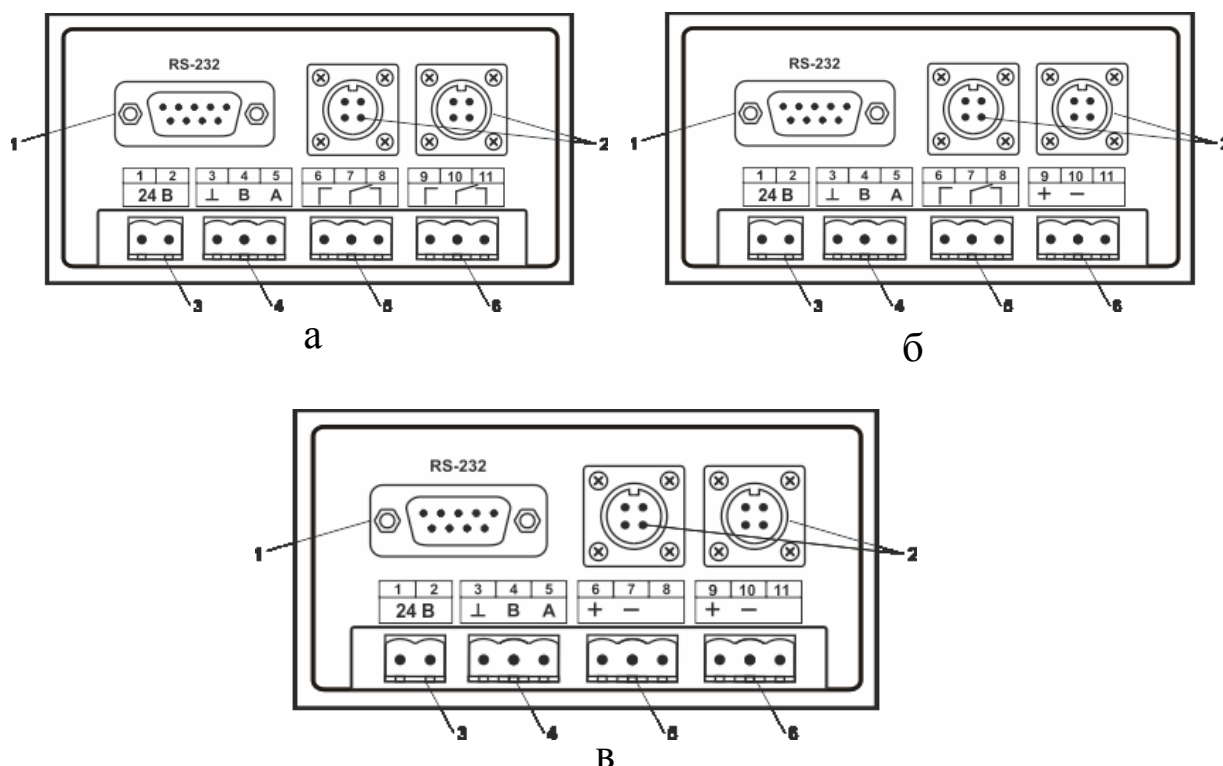
Рисунок 3.2 Задняя панель газоанализатора
