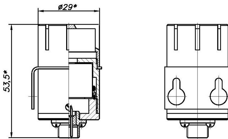
Рисунок 3.8 Преобразователь ИПК-01
