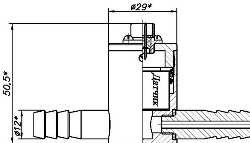
Рисунок 3.9 Преобразователь ИПК-02
