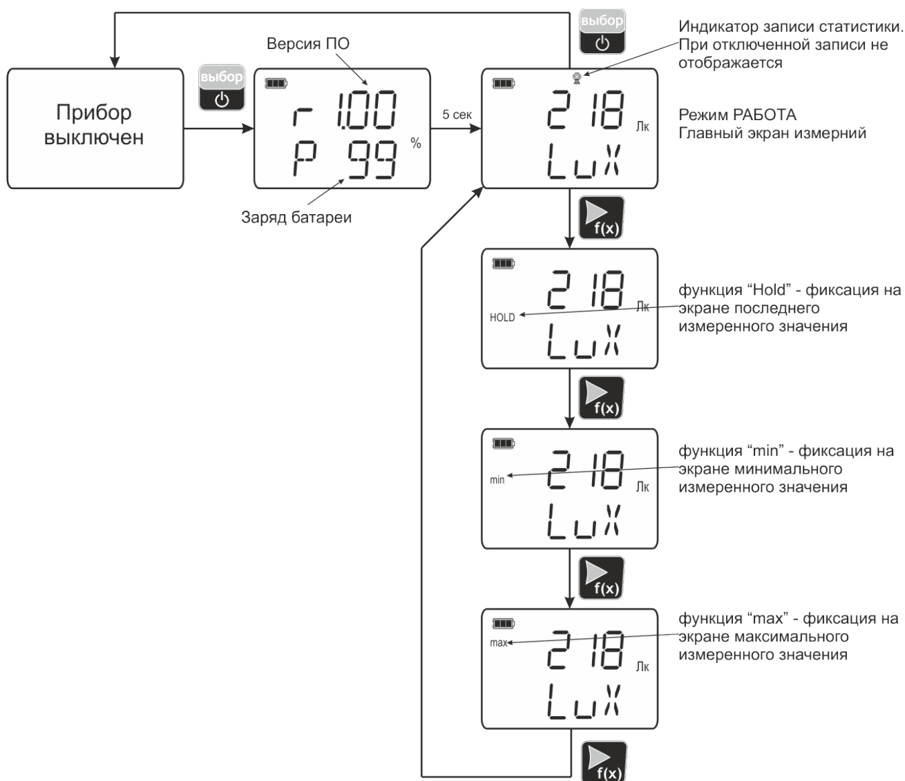
Рисунок 5.3 Схема режима РАБОТА люксметра ЛМ-12
