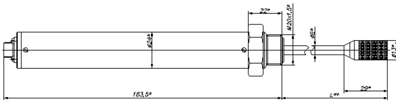
Рисунок Б5 Прибор ИВТМ-7 Н-06-ПВ(-ПС)
