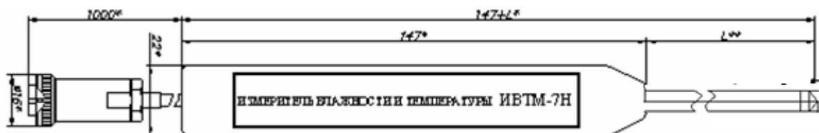
Рисунок Б4 Прибор ИВТМ-7 Н-05-1В
